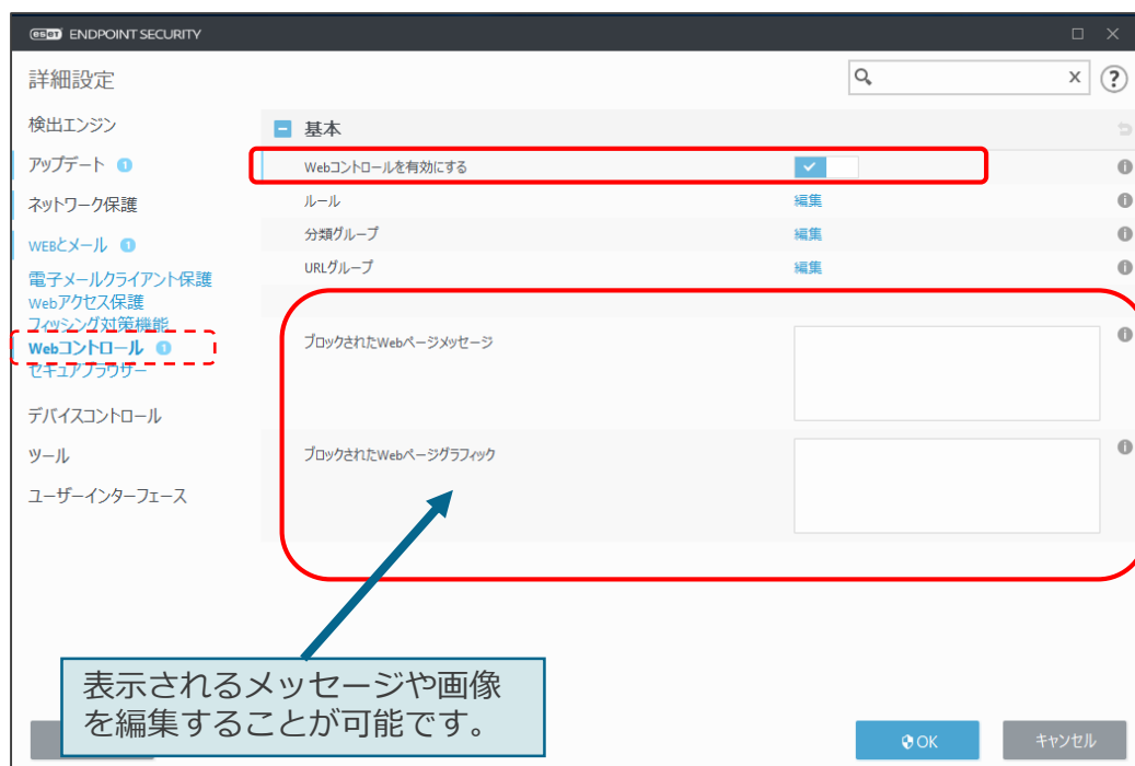
詳細設定(Webコントロール画面)
