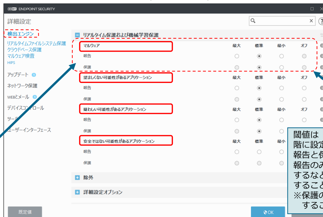
詳細設定(検出エンジン画面)
