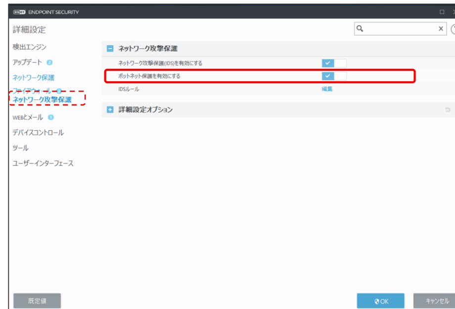
詳細検査(ネットワーク攻撃保護画面)
