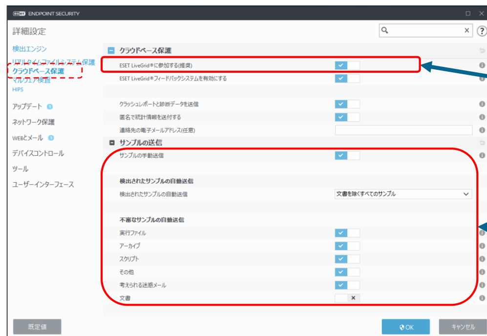
詳細設定(クラウドベース保護画面)
