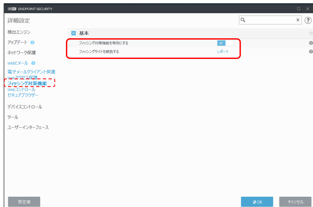
詳細設定(フィッシング対策機能画面)
